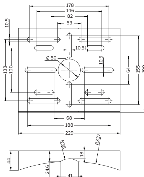
ESPECIFICACIONES DE BASE PARA MONTAJE DE MOTOR (mm)
